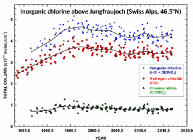
Figuur 3: Chloorreservoirs in de stratosfeer. Tijdreeksen van de maandelijkse gemiddelde hoeveelheden van de belangrijkste chloorreservoirs in de stratosfeer over meerdere decennia: waterstofchloride (HCl: rode cirkels) en chloornittraat ( \text{ClONO}_2 : groene driehoekjes) afgeleid uit infraroodwaarnemingen gerealiseerd vanuit het wetenschappelijk station in Jungfraujoch. De tijdreeksen zijn hier beperkt tot de maanden juni tot november, die gekenmerkt worden door kleinere atmosferische variaties. De twee reservoirmoleculen samen (blauwe driehoekjes) geven een goede indicatie van de evolutie van de totale hoeveelheid anorganisch chloor op gemiddelde breedtegraden in de noordelijke hemisfeer gedurende de laatste 30 jaar. (bron: GIRPAS – Universit  de Li ge, 2017)
