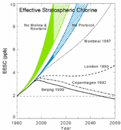
Figuur 2: Evolutie van EESC in ppb tussen 1980 en 2060 volgens de opeenvolgende aanpassingen aan het Montreal Protocol, en in de veronderstelling dat de productie van CFK's zou verdergezet zijn volgens het ritme van 1974 ('No Rowland en Molina') of volgens dat van 1987 ('No Montreal Protocol'). (bron: G. Velders, RIVM)
